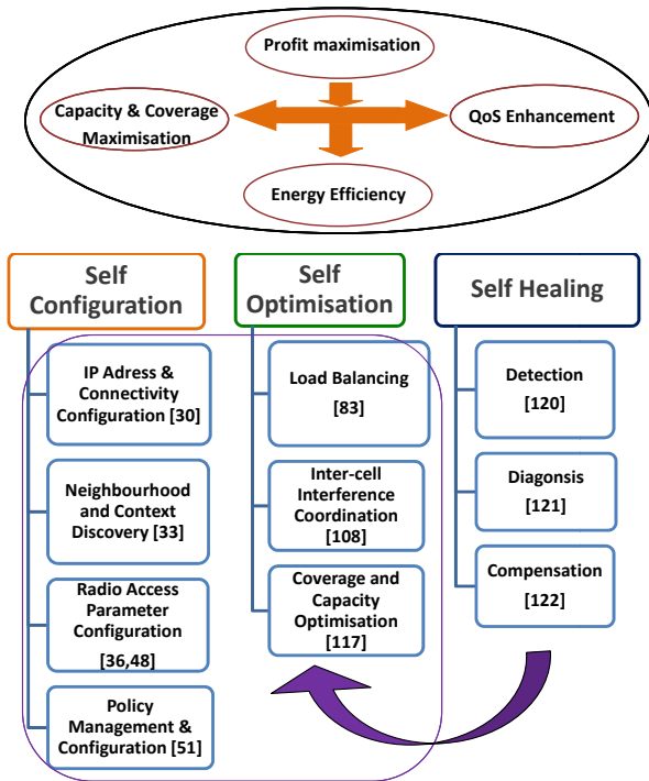
Fig. 1. SON Taxonomy
